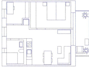
Schematische Apartmenteinheit für 2 Personen, mit Balkon, ca. 50,0m², o.M.
