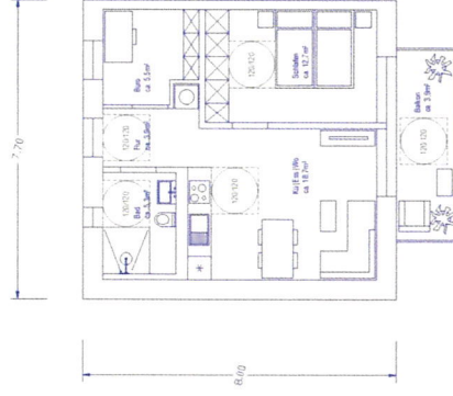
Schematische Apartmenteinheit für 2 Personen, ca. 50,0m², o.M.
